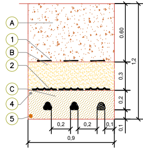
ZANJA MIXTA TIPO 2 (2T + 1BT)
