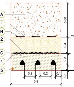
ZANJA TIPO 3 CIRCUITOS (3T-3C)
