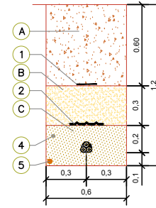
ZANJA TIPO BT (1 BT)
