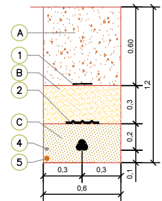
ZANJA TIPO 1 CIRCUITO (1T - 1C)
