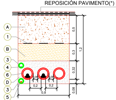
ZANJA TIPO 2 CIRCUITOS (CRUCE) (2T - 2C)
