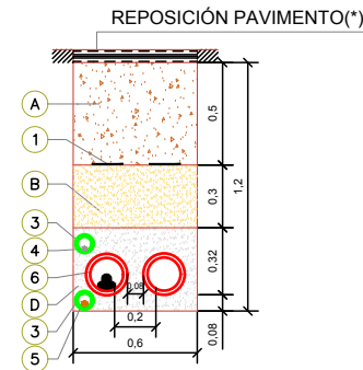
ZANJA TIPO 1 CIRCUITO (CRUCE) (1T - 1C)
