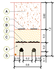
ZANJA MIXTA TIPO 1 (1T+1BT)
