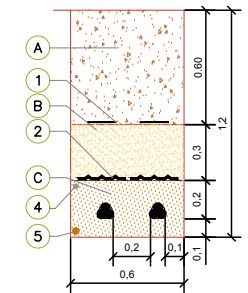
ZANJA TIPO 2 CIRCUITOS (2T - 2C)
