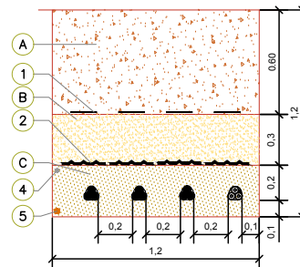
ZANJA MIXTA TIPO 3 (3T + 1BT)
